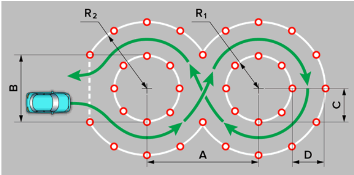
Схема 7. Позначення зони елемента "Вісімка"
