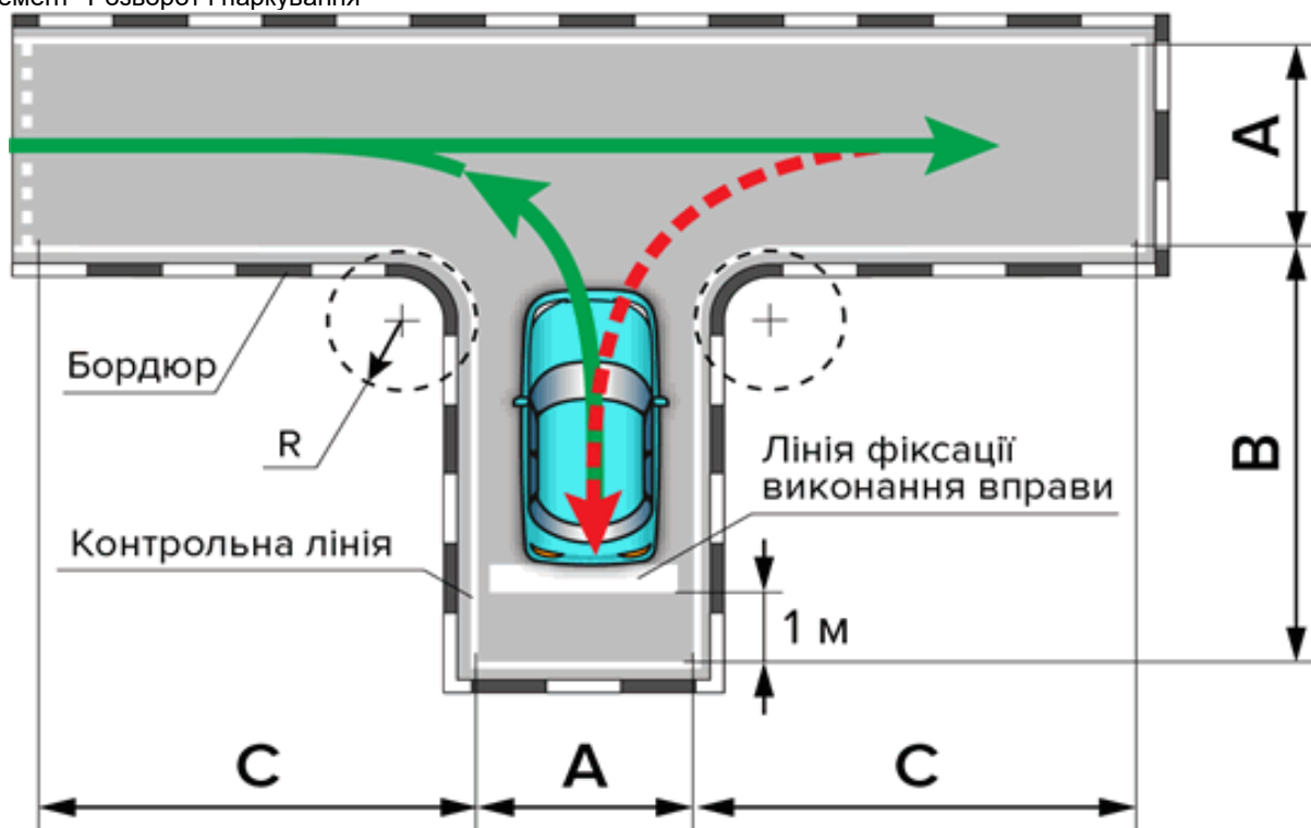
Схема 2. Позначення зони елемента "Розворот і паркування"
