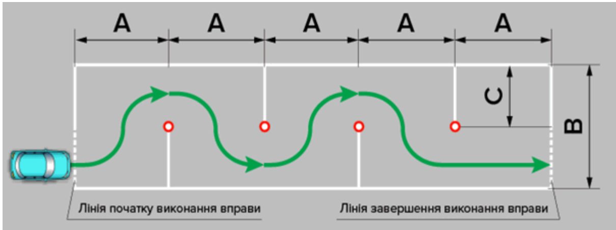
Схема 6. Позначення зони елемента "Змійка"
