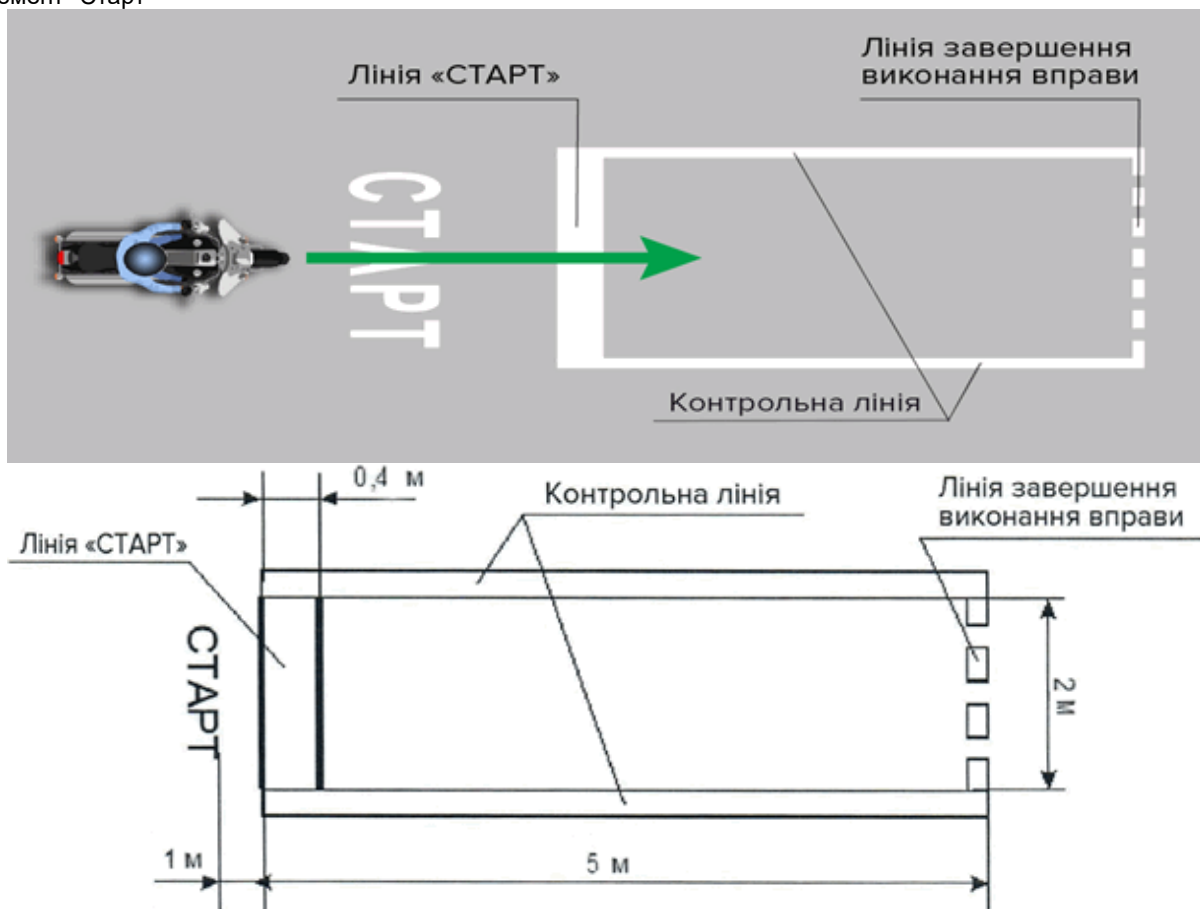
Схема 1. Позначення зони елемента "Старт"
