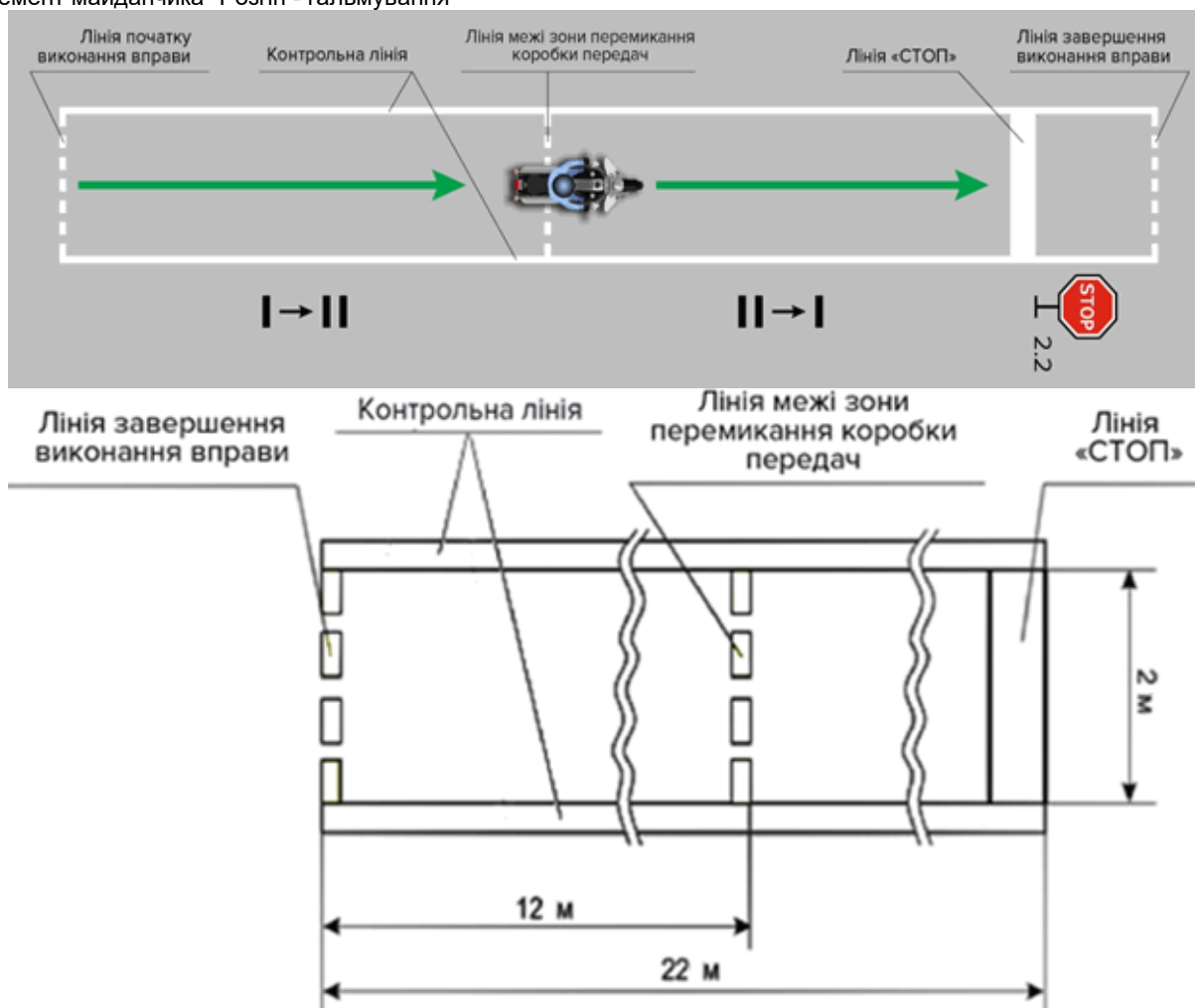
Схема 3. Позначення зони елемента "Розгін - гальмування"
