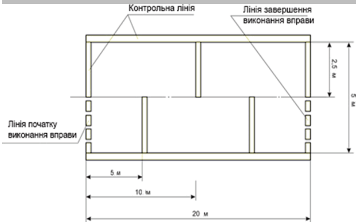
Схема 4. Позначення зони елемента "Змійка"
