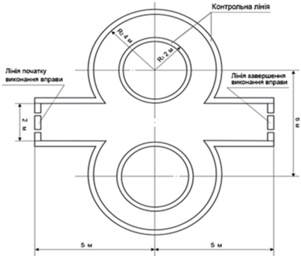
Схема 7. Позначення зони елемента "Вісімка"
