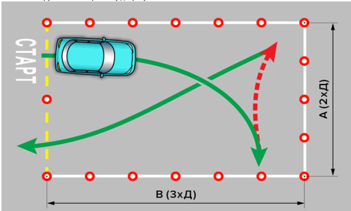
Схема 4. Позначення зони елемента "Маневрування в габаритному дворіку"
