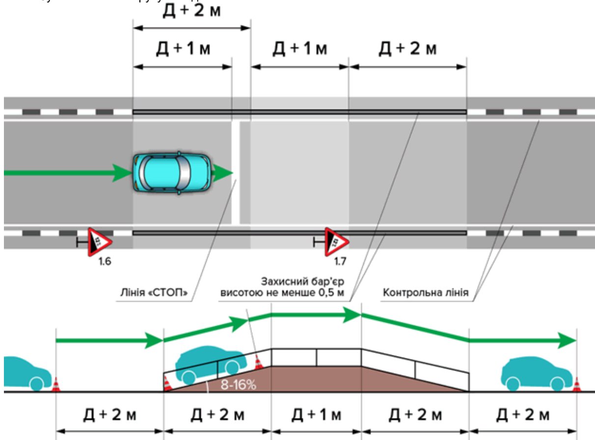
Схема 5. Позначення зони елемента "Зупинка і початок руху на підйомі"
