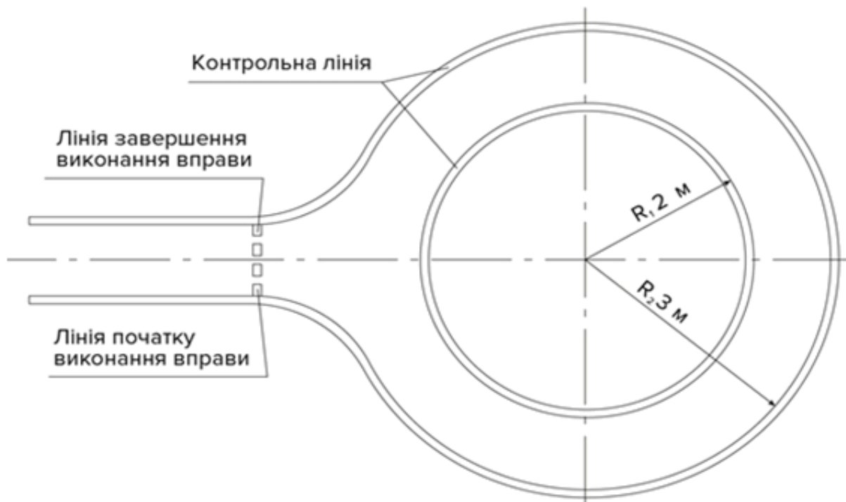
Схема 2. Позначення зони елемента "Коло"
